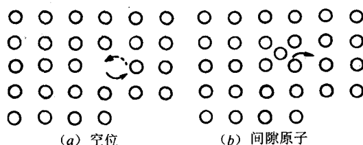
图 12-15 (a) 空位和(b) 间隙原子
