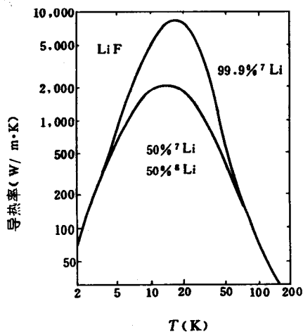
图 3-32 热导与杂质
