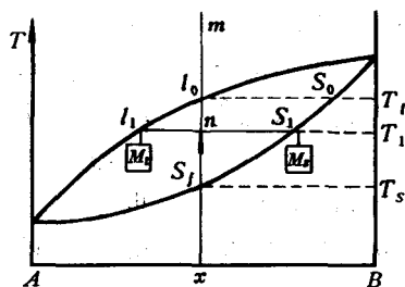
图 13-9 连续固溶体相图及其相变过程
