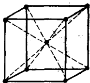
图 1-3 体心立方晶格的 典型单元
