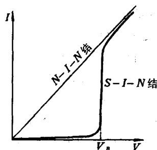
图 10-20 单粒子隧道效应的 电流-电压关系
