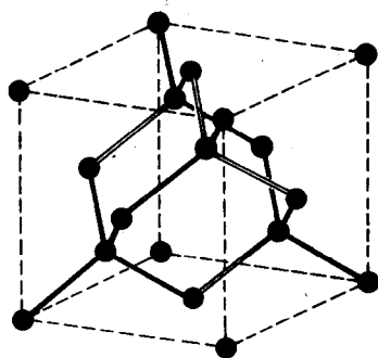
图1-8 金刚石晶格结构的典型单元
