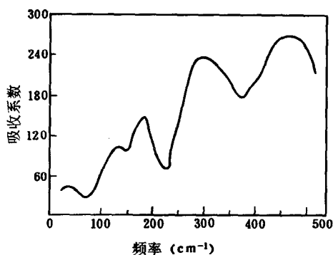
图 3-37 非晶硅的红外吸收光谱
