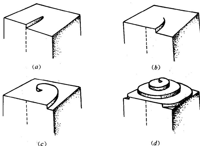
图 12-9 生长台阶的发展
