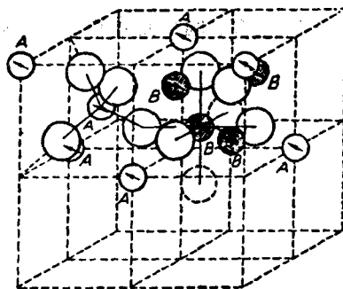
图 8-27 尖晶石结构
