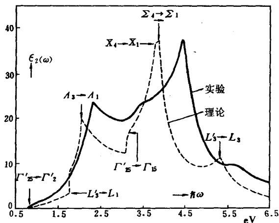
图 9-3 锆的介电常数的虚部; 实线: 实验结果; 虚线: 理论计算结果
