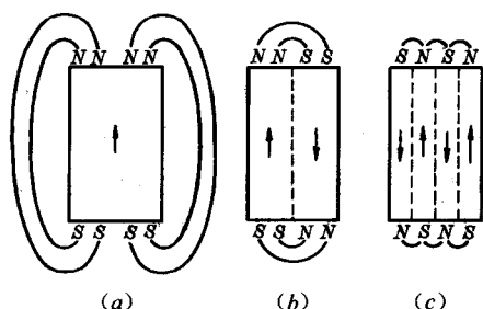
图 8-18 磁畴的分割和静磁能
