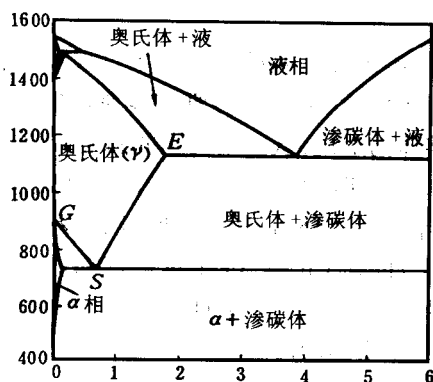
图 13-6 Fe-C 相图
