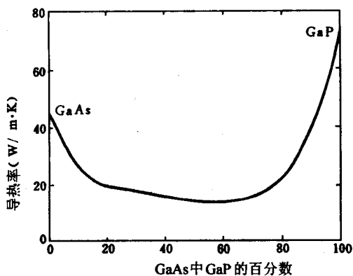
图 3-33 合金的热导
