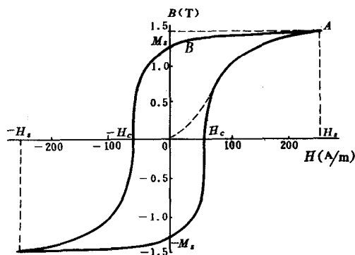
图 8-6 磁化曲线
