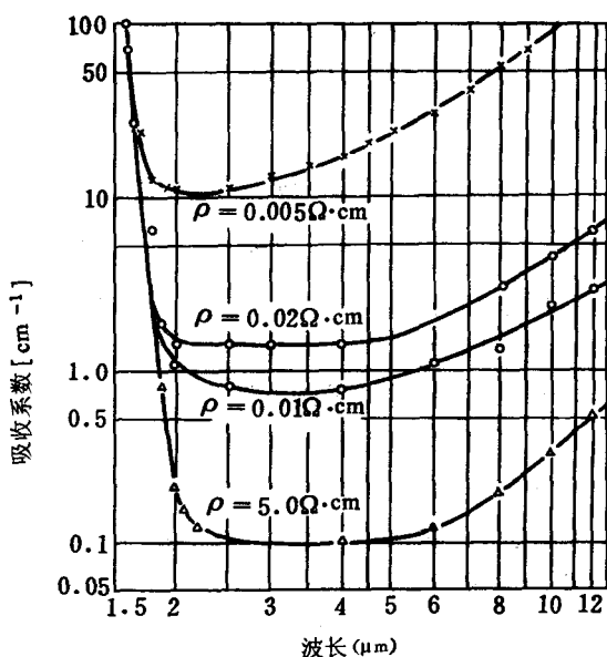
图 9-7 N 型锗的自由载流子吸收
