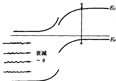
图 7-23 异质结的窗口效应
