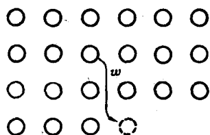
图 12-17 形成空位的示意图
