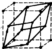
图 1-13 面心立方晶格的原胞
