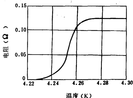
图 10-1 Hg 的电阻在低温下的变化
