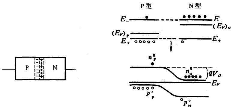
图 7-13 PN 结势垒
