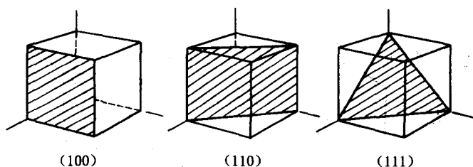
图 1-21 立方晶格中的(100)、(110)、(111)面
