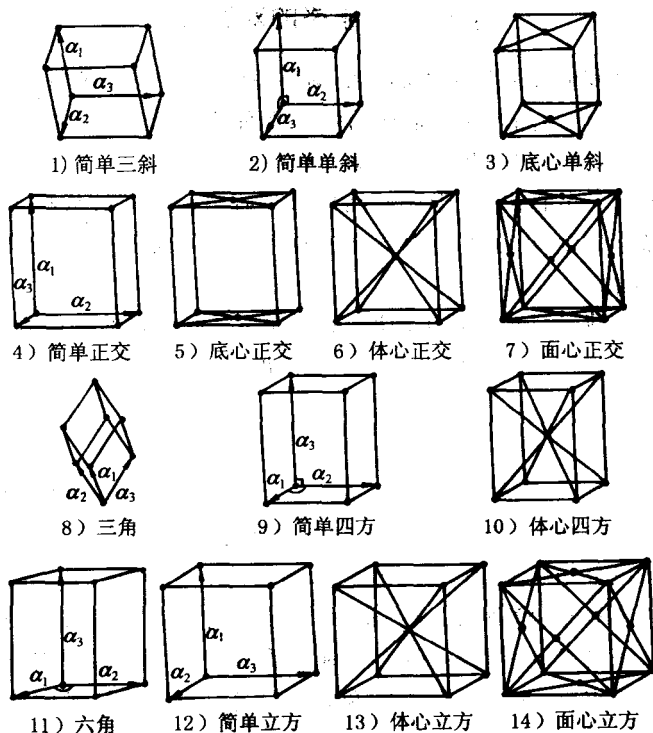
图 1-34 14 种布拉伐格子
