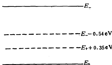
图 7-5 硅中金能级
