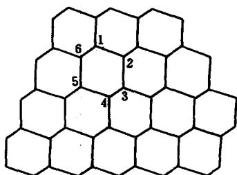
图 1-38 金刚石结构中的六原子环
