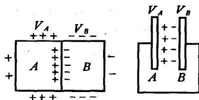
图 6-10 接触电势
