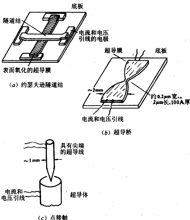
图 10-24 典型的弱连接超导体
