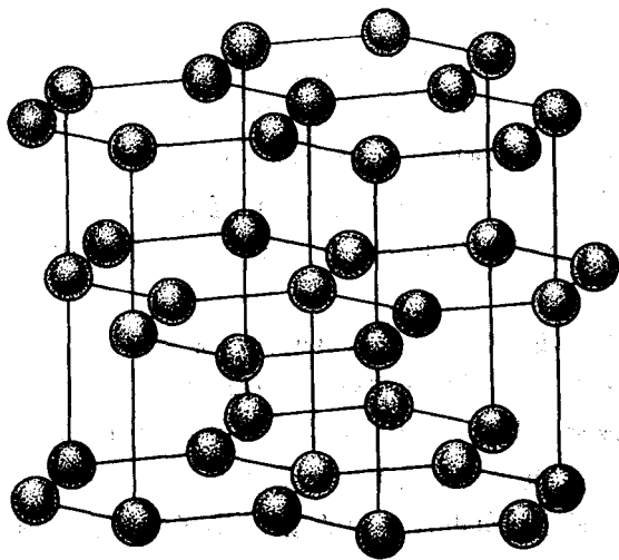
图 2-11 石墨晶格结构
