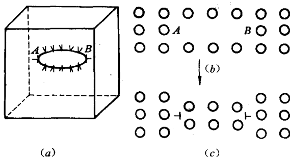
图 12-13 空位凝结和位错环
