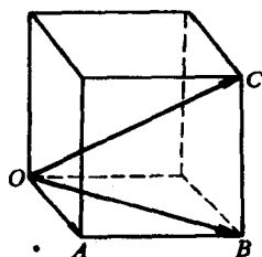
图 1-17 立方晶格中的 [100] 、 [110] 、 [111] 晶向
