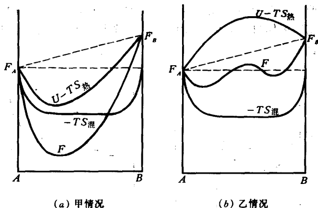
图 13-15 自由能曲线
