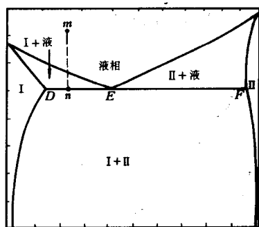
图 13-11 共晶转变
