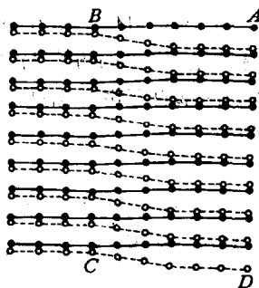
图 12-8 螺位错原子排列图
