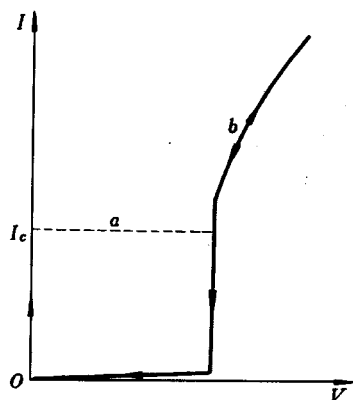
图 10-25 直流约瑟夫森效应的 电流-电压关系
