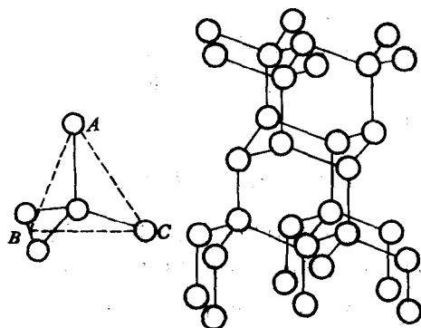
图 1-37 金刚石晶格的四面体单元及其网络
