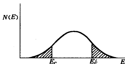
图 4-51 非晶态材料的能态密度
