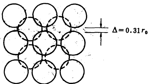
图 1-4 体心立方晶格的堆积方式
