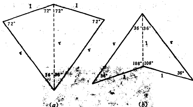
图 1-41 “箭”和“风筝”四边形
