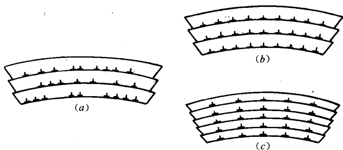
图 12-12 弯曲晶体中的位错排列
