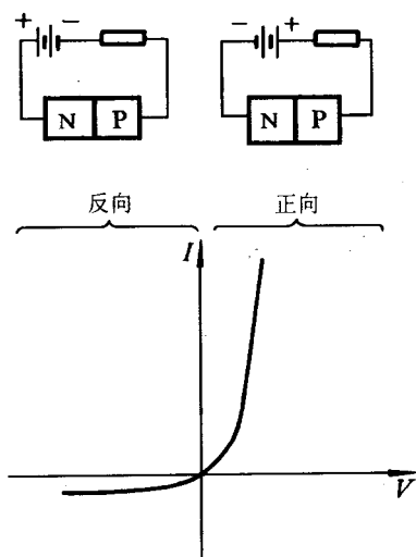
图 7-12 PN 结的单向导电性
