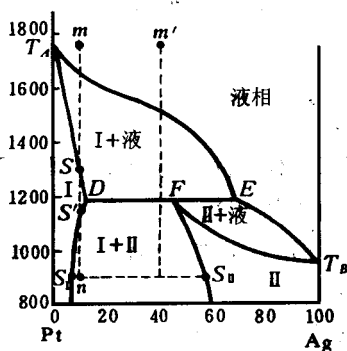
图 13-3 Pt-Ag 相图
