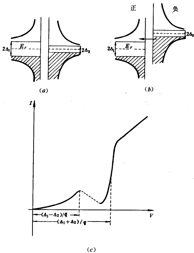
图 10-23 S-I-S 结的单粒子隧道电流
