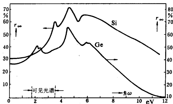
图 9-2 硅和锗在室温下的反射系数
