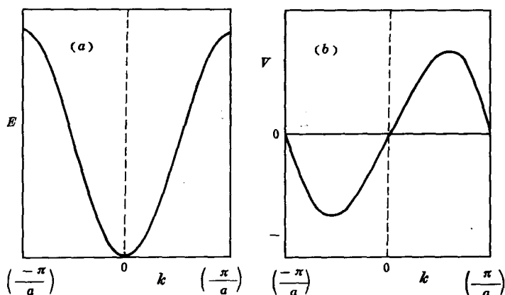
图 5-2 一维周期场中运动的电子的速度
