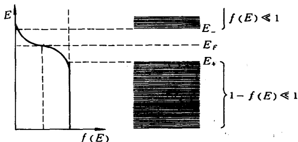
图 7-6 费米分布函数
