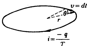
图 8-2 轨道运动的面积速度
