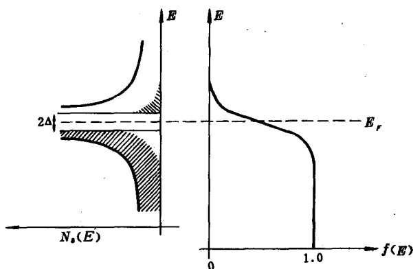
图 10-21 超导态的单粒子态密度, 以及在 T \approx 0K 时, 电子的分布
