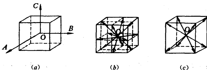
图 1-26 立方晶格中的对称轴
