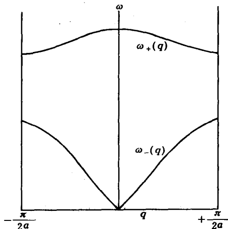
图 3-6 声学波和光学波
