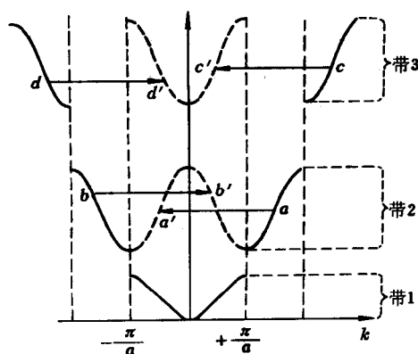
图 4-6 k 与简约波数 \bar{k} 之间的关系
