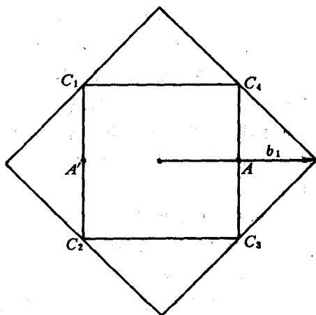
图 4-9 简单立方晶格中的简并态
