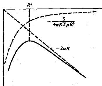
图 7-31 变程跳跃导电中的最可几的 R^*
