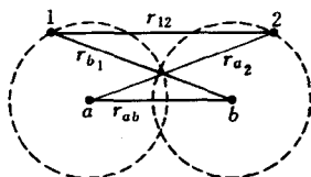
图 8-10 氢分子
