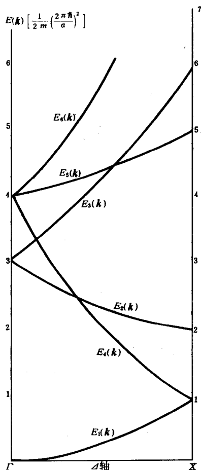
图 4-14 沿 \Delta 轴的自由电子的 E(k) 函数
