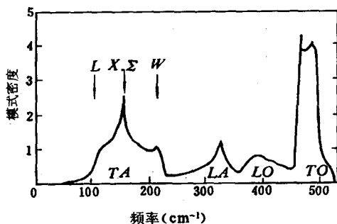
图 3-34 晶体硅的模式密度
