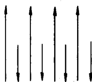
亚铁磁性
