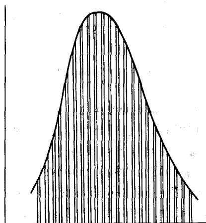
图 9-9 多声子谱包络
