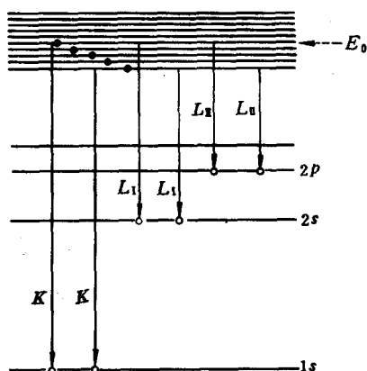
图 4-46 X 射线发射的能级图
