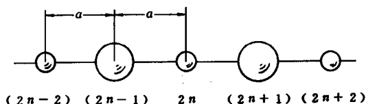
图 3-5 一维双原子链模型
