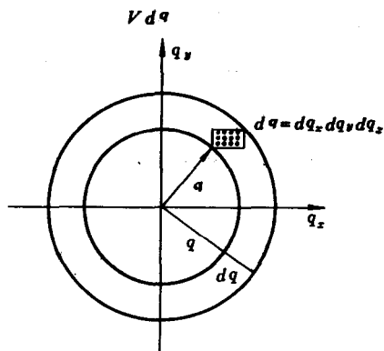
图 3-22 振动模在 k 空间的分布
