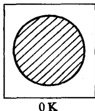
图 6-2 费米面和热激发
