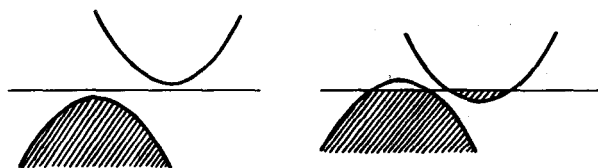
图 6-20 Wilson 转变的示意图
