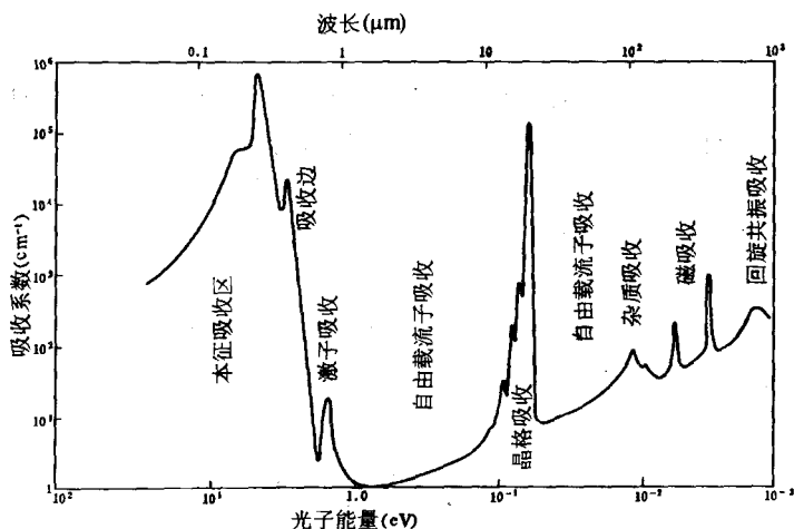
图 9-1 一个设想的半导体吸收光谱
