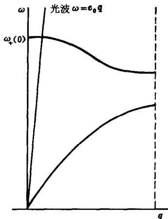
图 3-8 电磁波和光学波的共振
