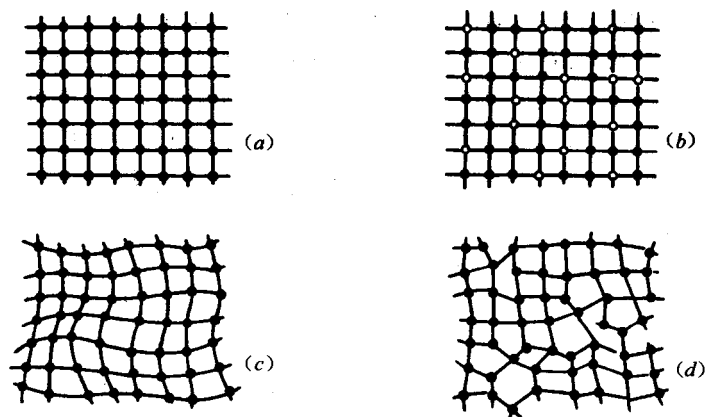
图 4-49 典型的无序类型
