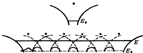
图 4-1 一维周期场
