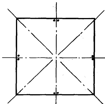
图 4-31 二维正方晶格的 k 星
