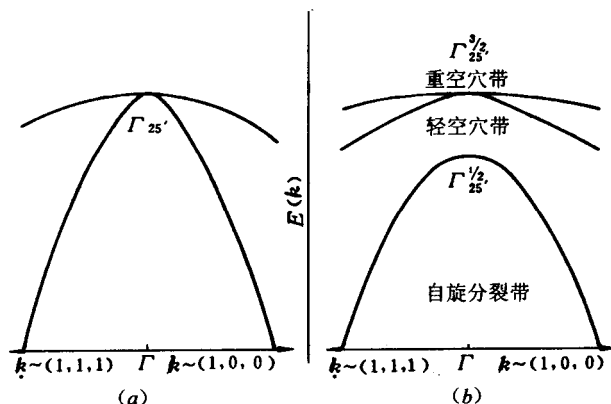
图 7-2 锗、硅价带结构示意图
