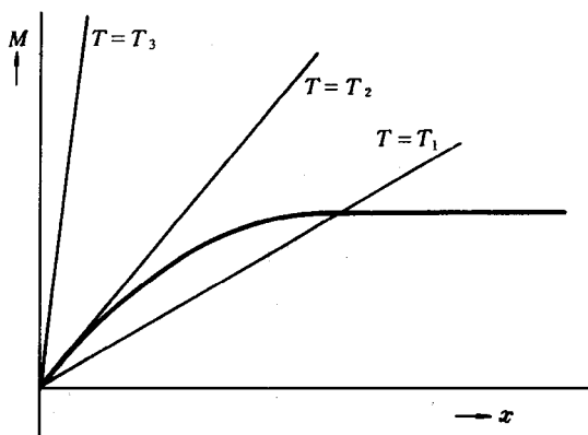
图 8-7 自发磁化图解
