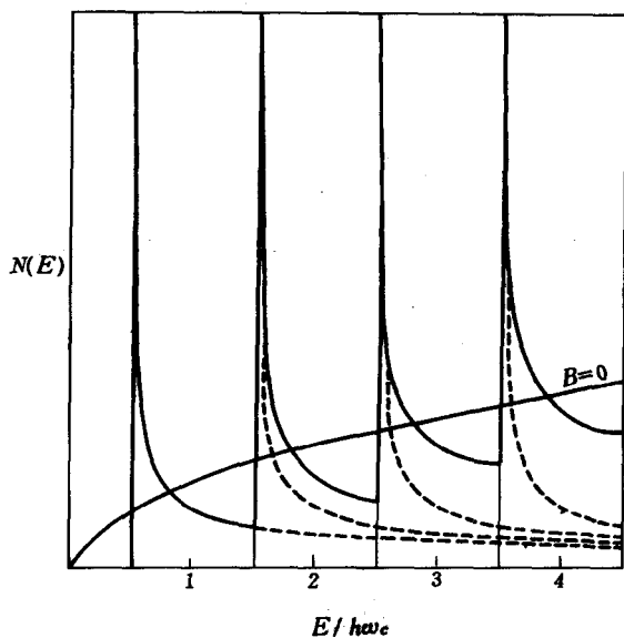
图 5-24 磁场中自由电子气的能态密度
