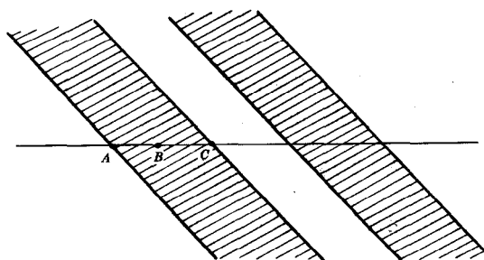
图 5-6 电场作用下电子在实空间的运动
