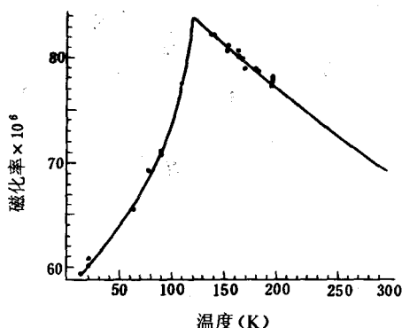
图 8-25 反铁磁体 MnO 的磁化率和温度
