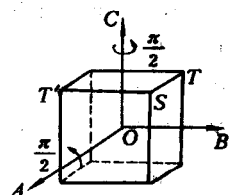
图 1-30 连续进行对称操作的实例
