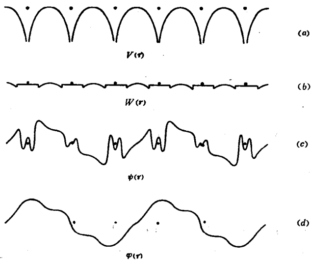
图 4-20 变势方法的示意图
