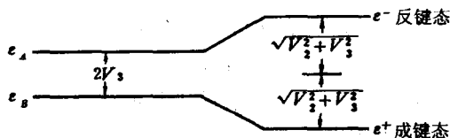
图 2-5 两个不同种原子的成键态和反键态
