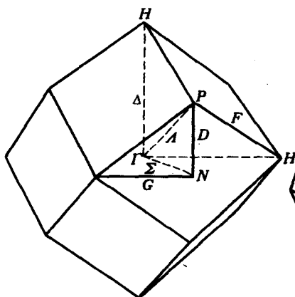
图 4-12 体心立方晶格的简约布里渊区
