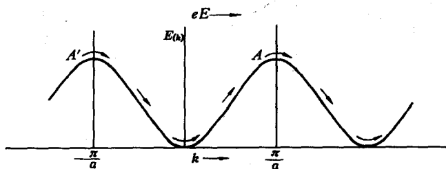
图 5-4 电子在恒定电场作用下的运动
