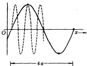
图 3-2 格波 q 的不唯一性的图示
