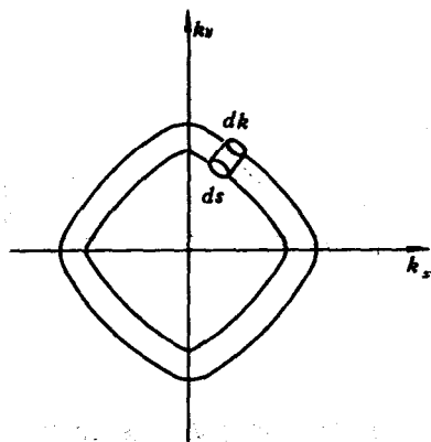
图 4-36 k 空间的等能面示意图
