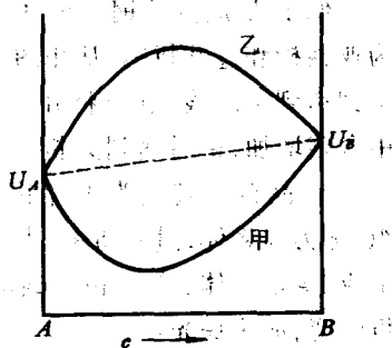
图 13-14 能量函数的两种情况
