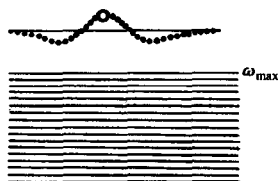
图 3-17 晶格振动的局域模
