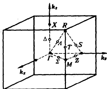
图 4-24 简单立方布里渊区
