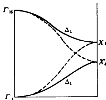
图 4-29 s 能带与 p 能带的交叠
