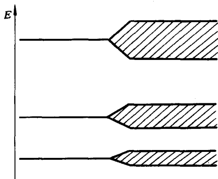
图 4-28 原子能级与能带之间的对应
