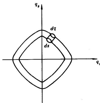
图 3-26 等频面示意图
