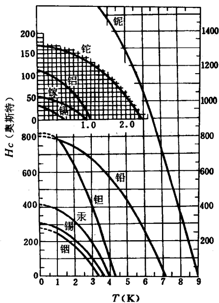
图 10-5 临界场和温度
