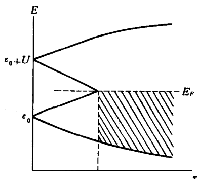
图 6-22 上、下 Hubbard 带及其交叠
