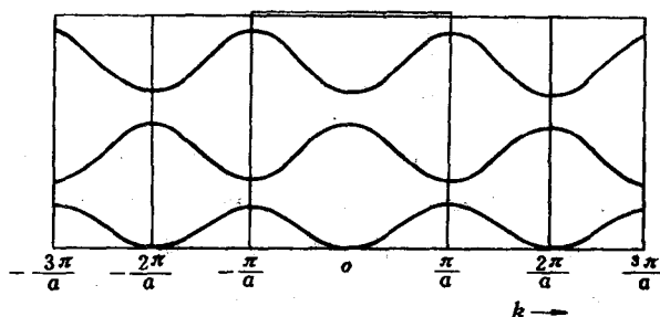
图 4-32 周期布里渊区图象
