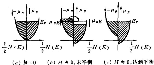
图 8-4 电子自旋顺磁性的分析
