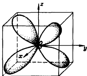
图 2-4 碳原子的杂化轨道
