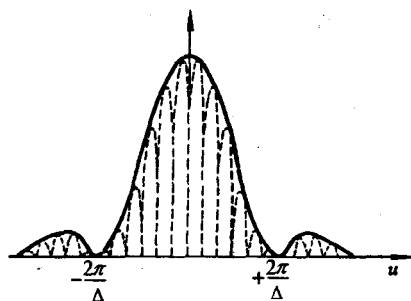
图 5-1 波包
