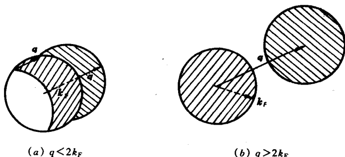
图 11-1 单电子激发
