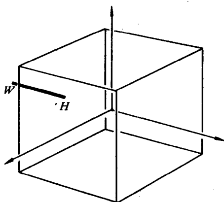
图 4-17 k 空间示意图
