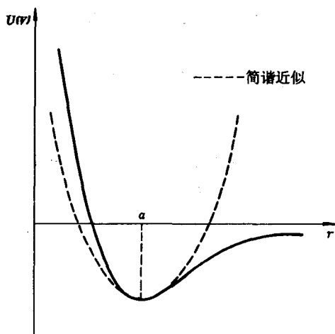
图 3-28 势能曲线图, 虚线表示简谐近似
