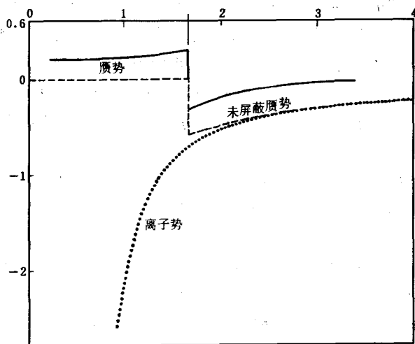
图 4-22 金属钠根据空中心模型的赝势
