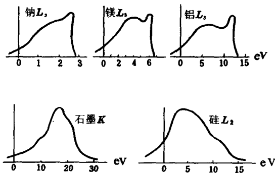
图 4-47 典型 X 射线发射谱
