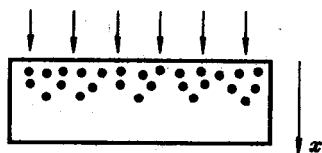
图 7-11 光产生的非平衡载流子分布
