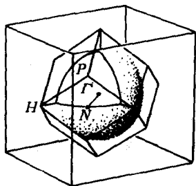
图 5-25 碱金属的费米面
