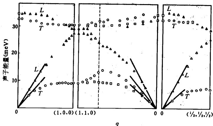
图 3-11 GaAs 的格波谱
