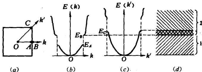
图 4-11 能带间的交叠
