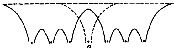
图 4-23 U(\xi) - V(\xi) 示意图
