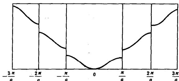
图 4-33 扩展布里渊区图象
