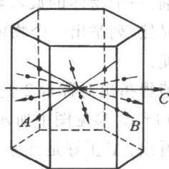
图 1-28 六角密排晶格中的对称轴
