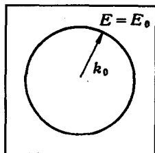
图 4-44 费米球
