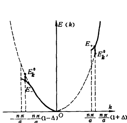
图 4-3 能量的微扰
