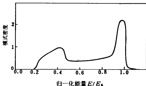
图 3-35 非晶硅的模式密度
