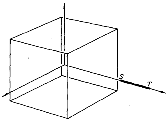
图 4-19 k 空间示意图
