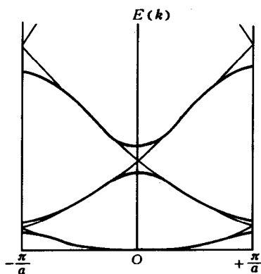
图 4-7 近自由电子近似的简约波数表示
