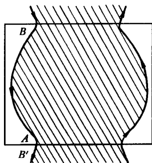
图 5-28 开轨道
