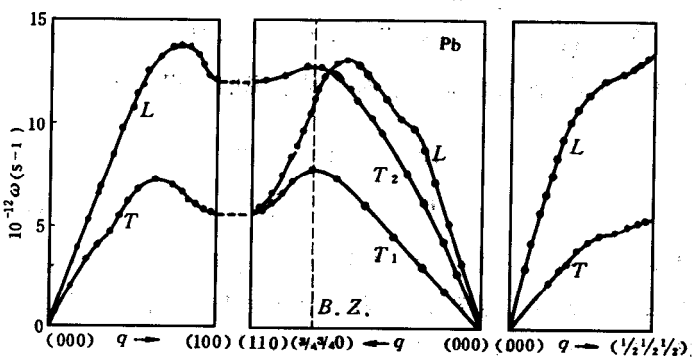
图 3-12 Pb 的格波谱
