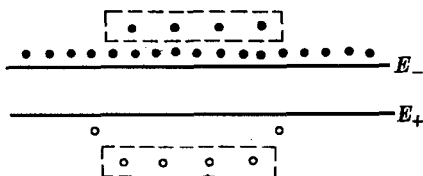
图 7-10 非平衡载流子示意图
