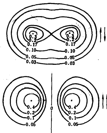
图 2-2 H_2 分子中电子云的等密度线图
