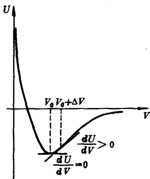
图 3-27 热膨胀示意图
