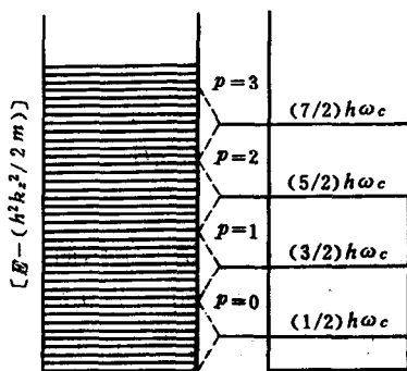
图 5-20 朗道能级的简并度
