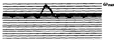
图 3-18 晶格振动的共振模
