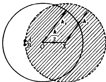
图 10-14 载流超导体的动量分布
