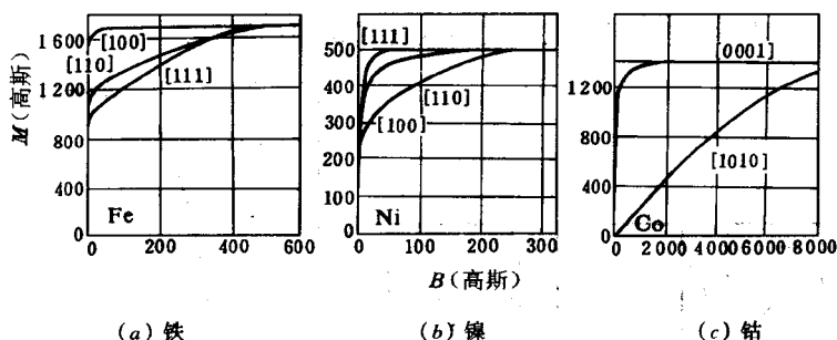
图 8-19 磁化的各向异性
