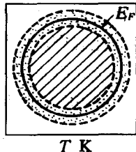
图 6-2 费米面和热激发
