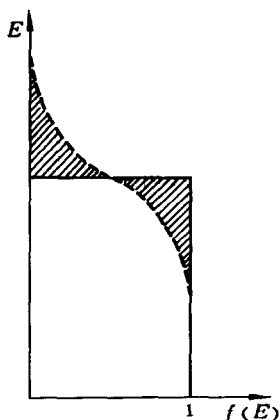
图 6-5 费米分布函数
