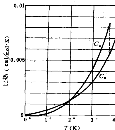
图 10-7 锡的比热曲线
