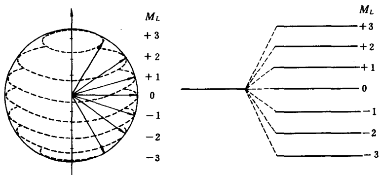
图 8-1 磁场中的塞曼分裂
