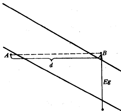
图 5-7 隧道穿透中的位垒长度
