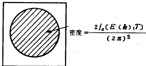
图 6-13 电子在 \mathbf{k} 空间的分布
