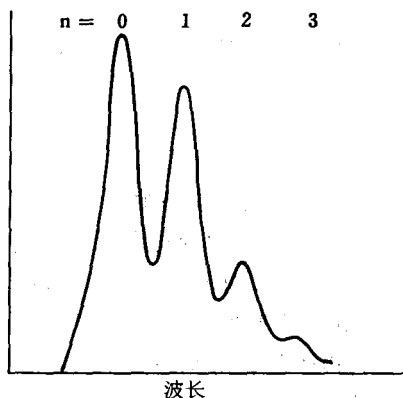
图 9-8 CdS 带边辐射
