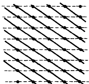
图 1-16 晶列
