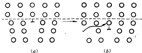
图 12-14 攀移
