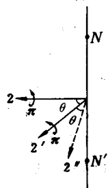
图1-33 两个二重轴之间的夹角
