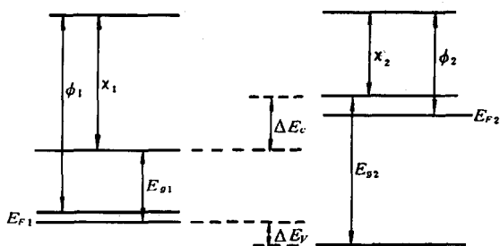
图 7-21 两种半导体材料的能带图
