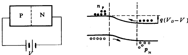
图 7-14 正向 PN 结势垒
