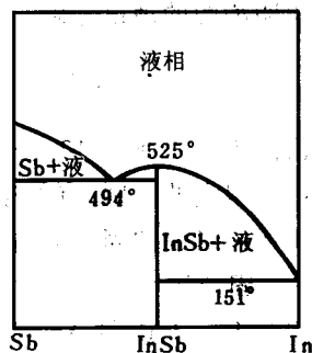
图 13-4 Sb-In 相图
