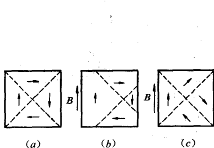
图 8-20 技术磁化机构
