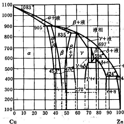
图 13-5 Cu-Zn 相图
