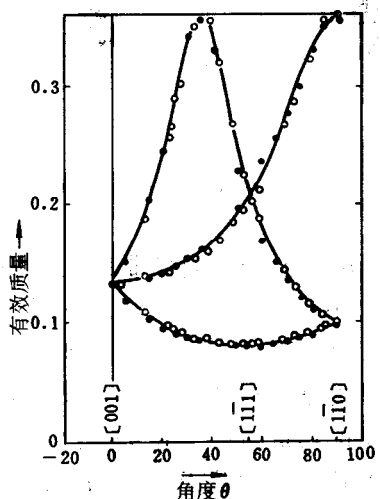
图 5-16 N 型锗回旋共振实验
