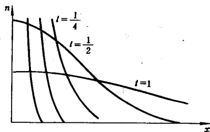
图 12-18 扩散分布
