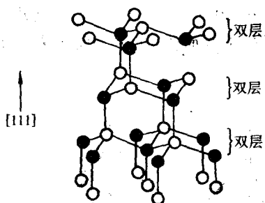
图 1-23 金刚石晶格中的双层密排面
