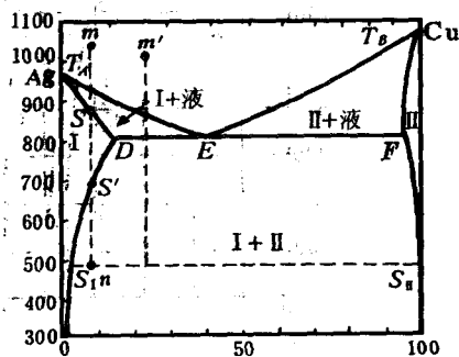
图 13-2 Ag-Cu 相图
