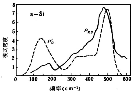
图 3-36 非晶硅的喇曼光谱
