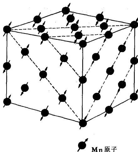
图 8-26 MnO 晶体反铁磁排列
