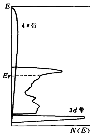
图 6-7 过渡金属能带
