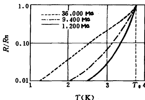
图 10-9 超导态和正常态表面电阻比值
