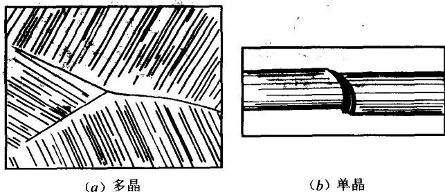
图 12-2 滑移带
