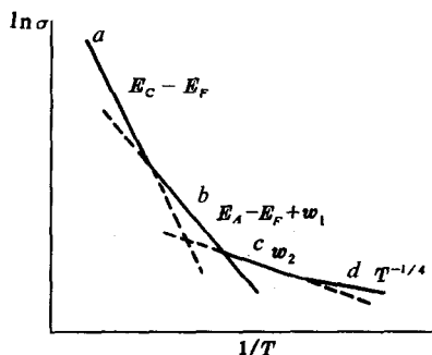
图 7-29 直流电导对温度的依赖关系
