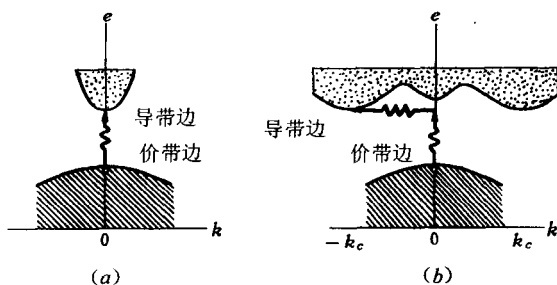
图 7-1 直接带隙(a)和间接带隙(b)
