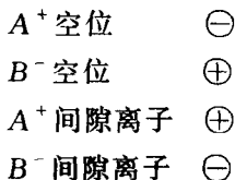
图 12-21 离子晶体中的缺陷
