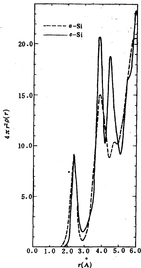
图 1-39 非晶硅和晶体硅的径向分布函数
