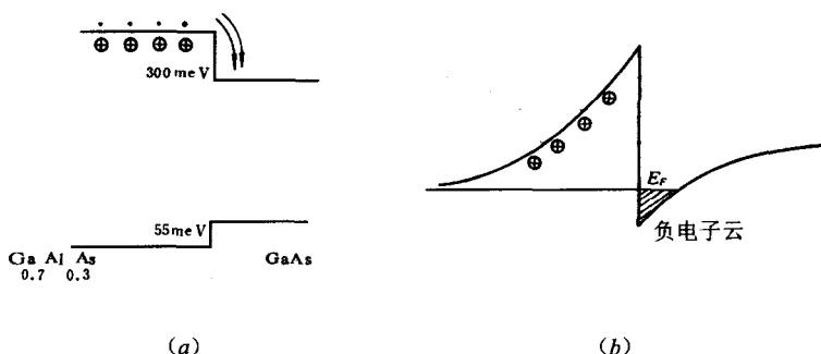
图 7-25 调制掺杂结构的能带图
