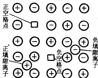
图 12-21 离子晶体中的缺陷
