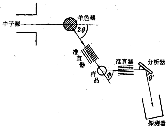
图 3-15 中子谱仪结构示意图
