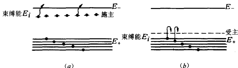
图 7-4 施主和受主电离能
