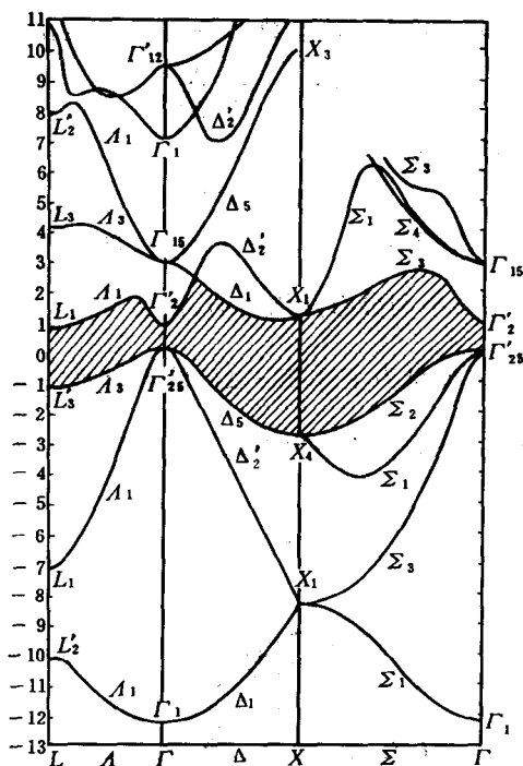
图 4-35 Ge 的能带
