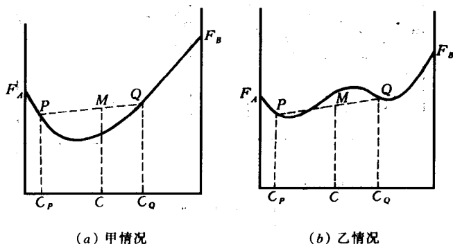
图 13-16 自由能曲线
