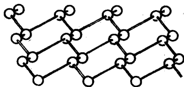
图 2-8 V 族元素 As、Sb 等的结构
