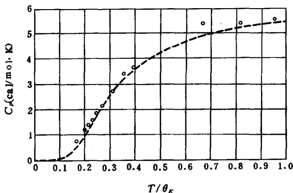
图 3-21 爱因斯坦理论与实验比较(圆点为金刚石实验值,温度以 \theta_E = \hbar\omega_0/k 为单位)
