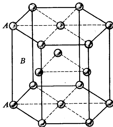
图 1-6 六角密排晶格的典型单元
