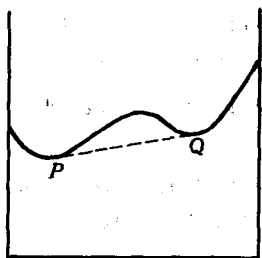
图 13-17 两相混合的自由能
