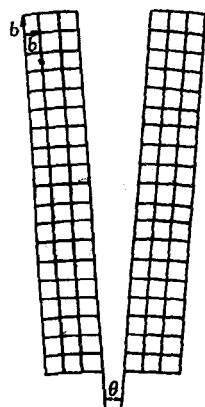
图 12-11 倾斜晶界
