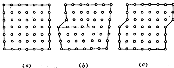
图 12-5 滑移过程图
