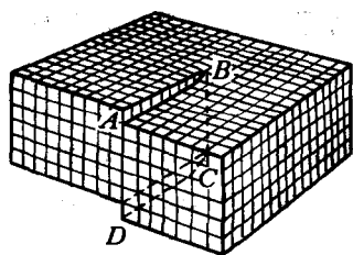
图 12-7 螺位错和滑移
