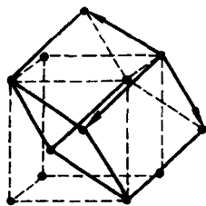
图 1-14 体心立方晶格的原胞
