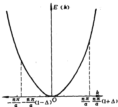
图 4-2 互相影响的状态
