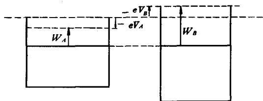
图 6-12 接触电势差和功函数
