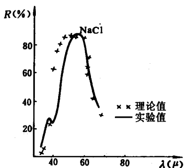
图 3-13 红外选择反射
