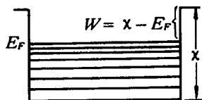
图 6-9 导带电子能量图
