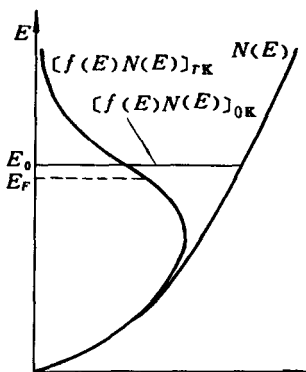
图 6-3 能态密度和电子按能量分布
