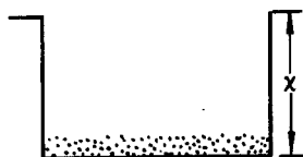
图 6-8 金属电子势阱
