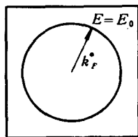
图 5-22 二维自由电子气的费米圆
