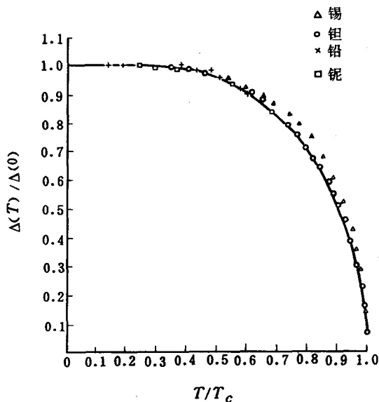
图 10-13 超导能隙随温度的变化
