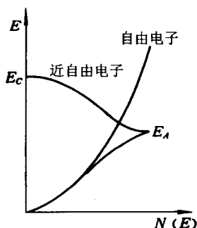
图 4-37 自由电子和近自由电子能态密度
