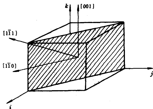
图 5-17 (110)面内磁场的变化示意图
