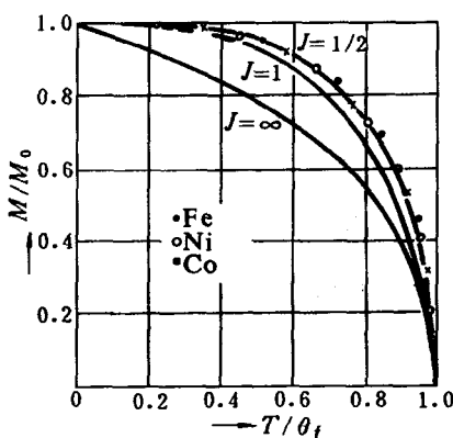
图 8-8 自发磁化和温度
