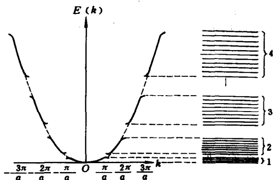
图 4-5 E(k) 图和能带
