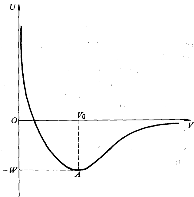
图 2-1 内能函数
