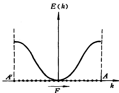
图 5-8 充满能带中的电子运动
