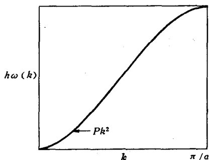
图 8-11 一维自旋波的色散关系
