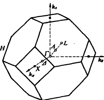
图 4-13 面心立方晶格的简约布里渊区
