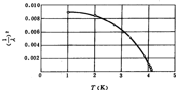
图 10-8 穿透深度和温度
