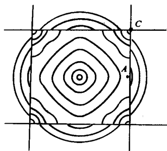
图 4-38 近自由电子等能面
