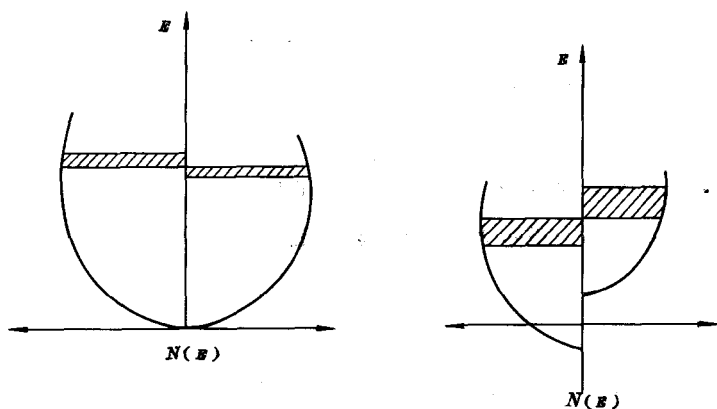
图 8-15 斯托纳模型
