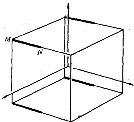
图 4-15 k 空间示意图
