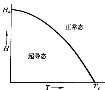
图 10-6 在磁场中的超导态和正常态
