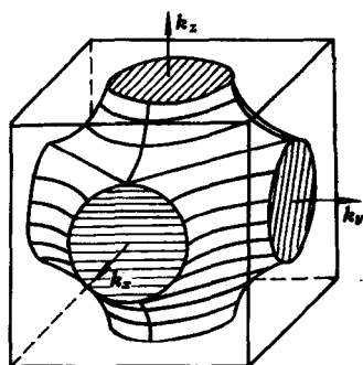
图 4-43 E = E_0 等能面
