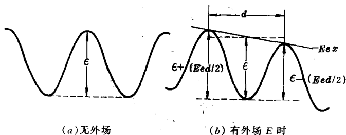
图 12-22 离子势能
