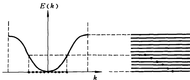
图 5-9 部分填充的能带
