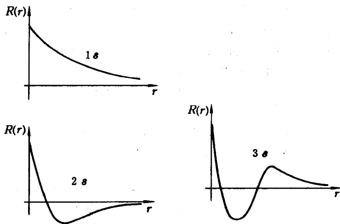
图 4-21 氢原子 1s 、 2s 、 3s 态的径向函数
