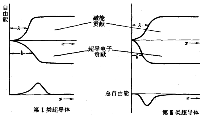
图 10-19 两类超导体的界面能的比较
