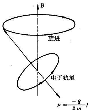
图 8-3 拉摩旋进
