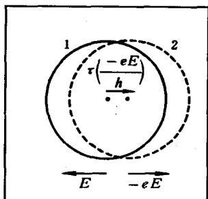
图 6-14 外场作用下的分布函数
