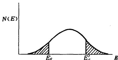
图 6-23 无序系统中的带尾定域态
