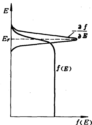
图 6-4 \left(-\frac{\partial f}{\partial E}\right) 的特点
