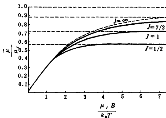
图 8-5 (\bar{\mu}/\mu_J) 随 \left(\frac{\mu_J B}{k_B T}\right) 的变化
