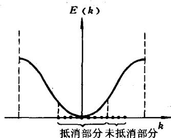
图 5-10 外场改变对称分布
