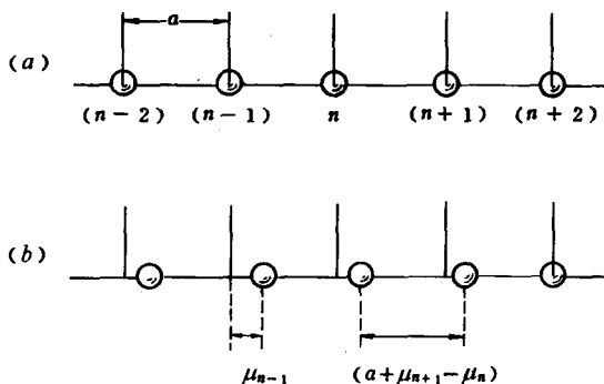
图 3-1 一维单原子链
