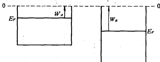
图 6-11 金属的能级图和功函数
