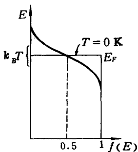
图 6-1 费米分布函数
