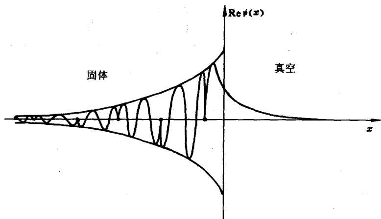
图 4-48 表面态波函数
