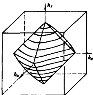
图 4-42 E = E_0 - 2J_1 等能面
