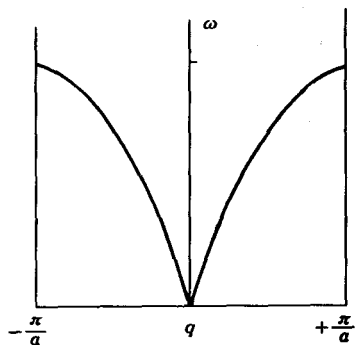
图 3-4 一维单原子链的 \omega - q 函数关系
