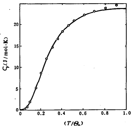
图 3-23 德拜理论与实验比较(实验点是锡的测量值)
