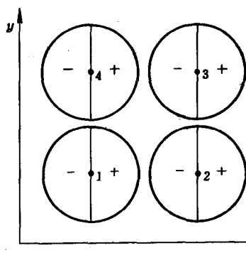
图 4-26 \varphi_{p_x} 原子波函数的正值和负数区域
