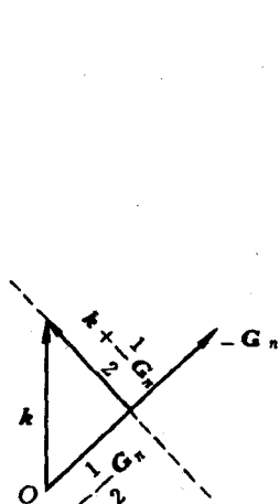
图 4-8 发散条件
