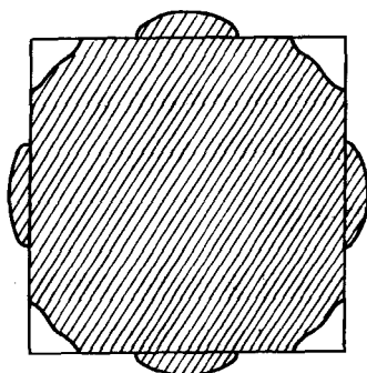
图 4-45 二价金属的费米面
