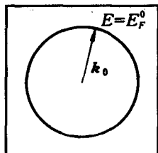
图 6-15 球形等能面
