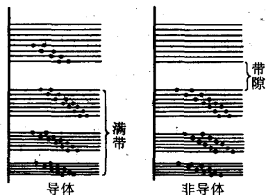
图 5-11 导体和非导体的能带模型
