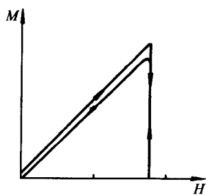
图 10-4 磁场中的超导转变
