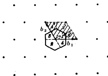
图 3-9 \mathbf{q} 的取值范围
