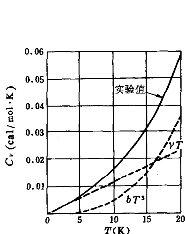
图 6-6 Fe 金属低温热容量
