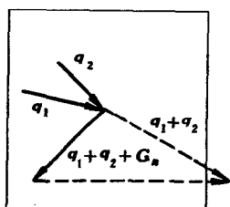
图 3-30 翻转过程
