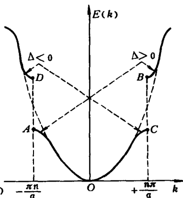
图 4-4 k = \pm \frac{n\pi}{a} 处的微扰
