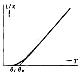
图 8-9 高温顺磁性
