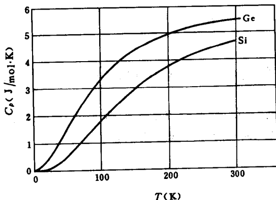
图 3-20 低温下晶格比热下降
