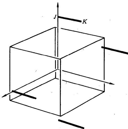
图 4-18 k 空间示意图
