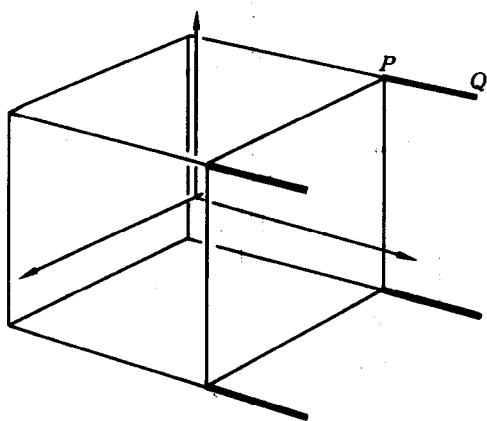
图 4-16 k 空间示意图
