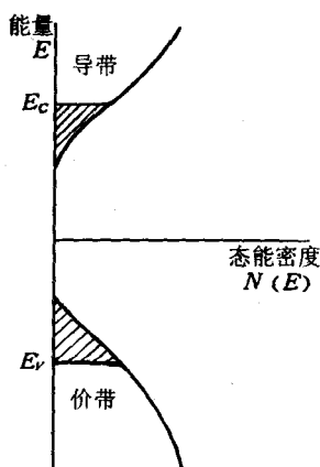
图 7-26 非晶态半导体的态能密度
