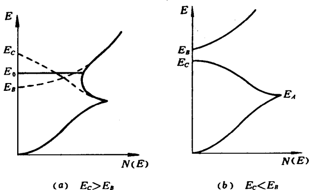
图 4-39 重叠和不重叠能带的能态密度
