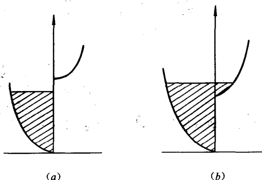
图 8-16 自发磁化的两种典型情况
