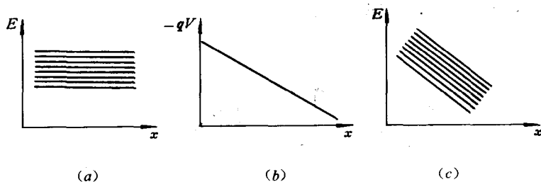
图 5-5 能带的倾斜
