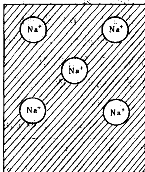
图 2-7 金属性结合示意图
