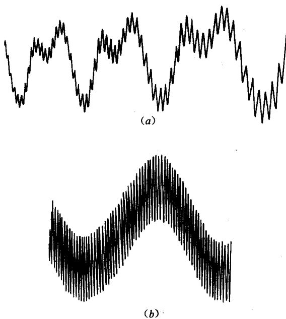
图 5-19 德·哈斯-范·阿芬效应 (a) 镉 (b) 银
