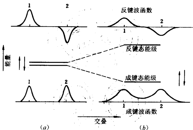
图 2-3 成键态和反键态
