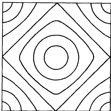
图 4-40 紧束缚近似等能面示意图
