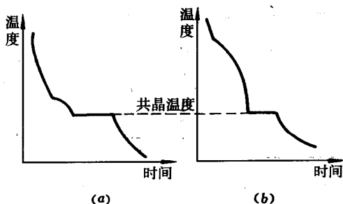
图 13-13 包含共晶转变的冷却曲线
