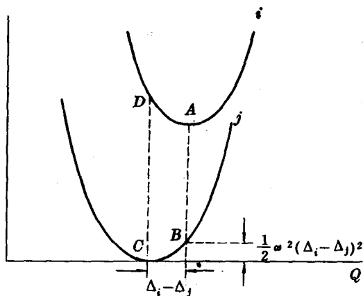
图 9-10 位形坐标图
