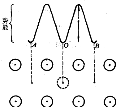
图 12-16 间隙原子的势垒
