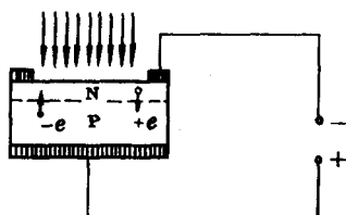
图 7-24 PN 结光生伏特效应
