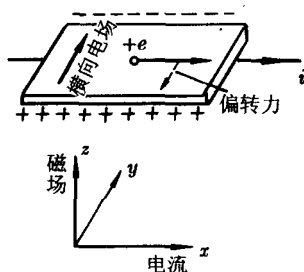
图 7-8 霍耳效应
