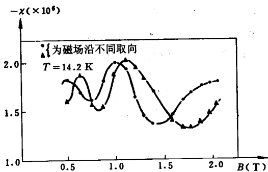
图 5-18 14.2K 镉单晶磁化率随磁场的变化
