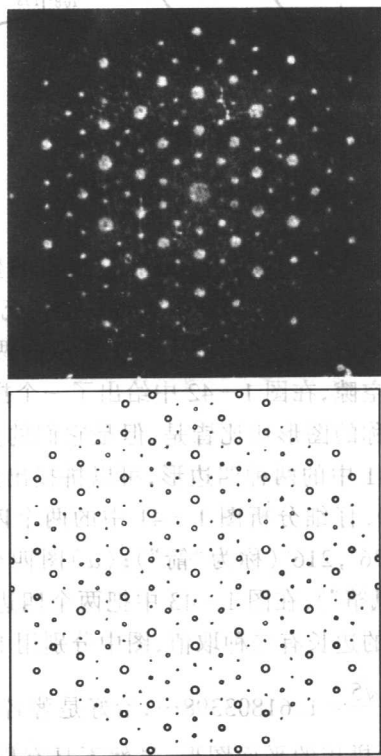
图 1-40 AlMn 合金的电子衍射图
