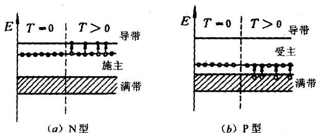
图 7-3 施主和受主
