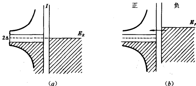
图 10-22 S-I-N 结单粒子隧道电流
