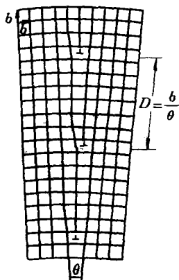
图 12-10 小角晶界
