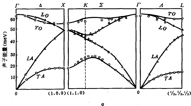
图 3-10 硅的格波谱
