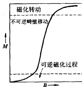
图 8-21 磁化过程的分析
