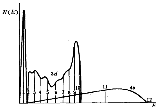
图 8-13 过渡金属中的 3d 和 4s 能带
