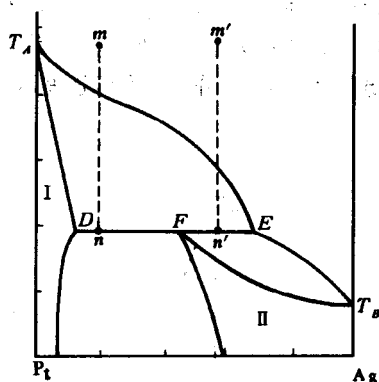
图 13-12 包晶转变
