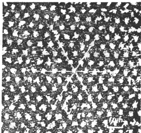
图 10-18 混合态结构的实验观察
