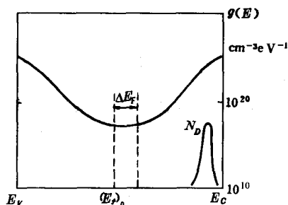
图 7-28 掺杂效应中缺陷态的影响
