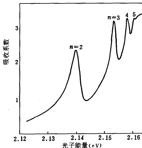
图 9-5 77K 下 \text{Cu}_2\text{O} 的激子吸收线
