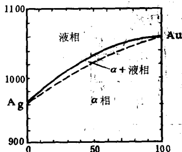
图 13-1 Ag-Au 相图
