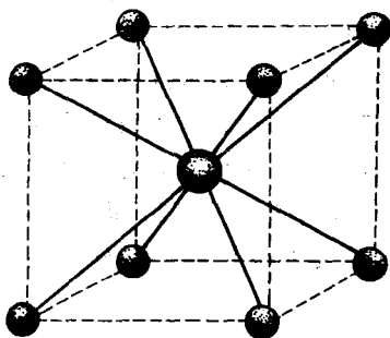
图 1-10 CsCl 晶格结构的典型单元
