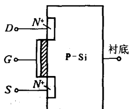
图 7-18 N 沟道 MOS 晶体管
