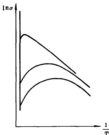
图 7-7 锗的电导率和温度关系
