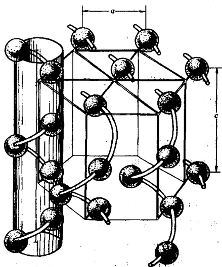
图 2-9 硒、碲的结构
