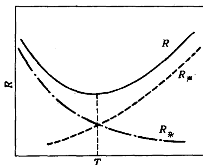
图 6-19 近藤效应示意图
