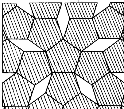
图1-32 晶格中不可能存在五重轴的示意图
