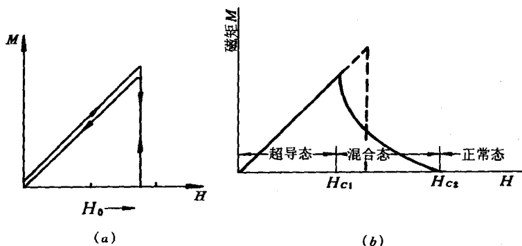
图 10-15 磁化曲线
