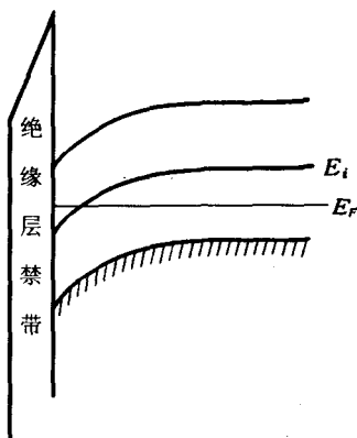
图 7-17 表面反型层能带图
