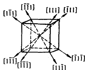
图 1-19 [111] 及其等效晶向
