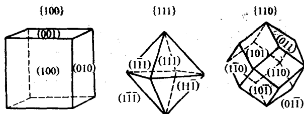
图 1-22 立方晶格中的等效晶面
