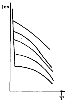
图 7-9 电子浓度与温度
