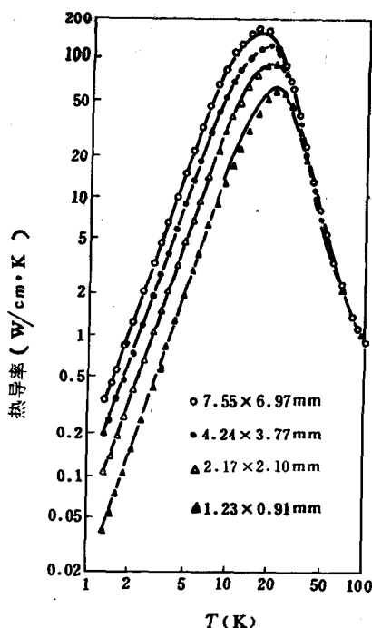
图 3-31 热导与样品尺寸之间的关系
