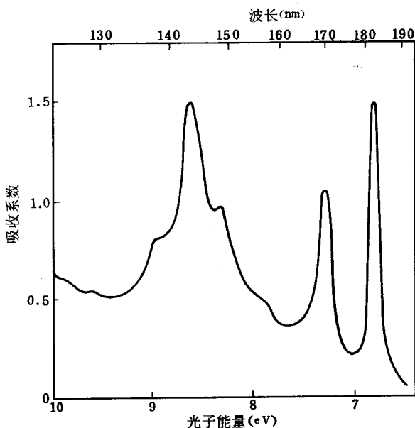
图 9-6 77K 下 KBr 的激子吸收谱线
